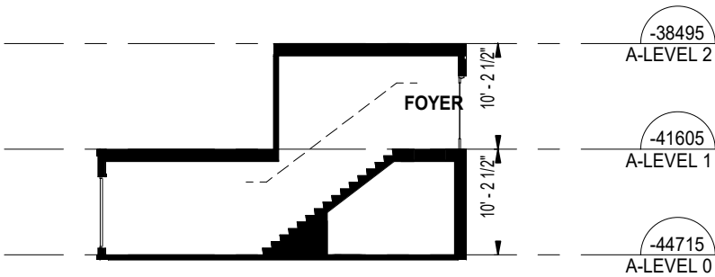
UNIT 030/070 - SECTION
