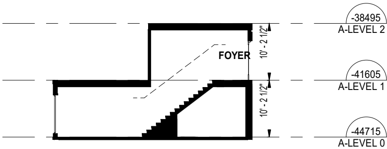
UNIT 020/060 - SECTION
